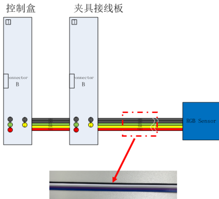
图 3-5 RGB 接线示意图
