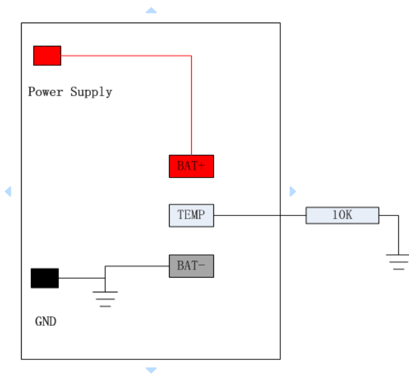
图 3-2 NTC 夹具接线方法
